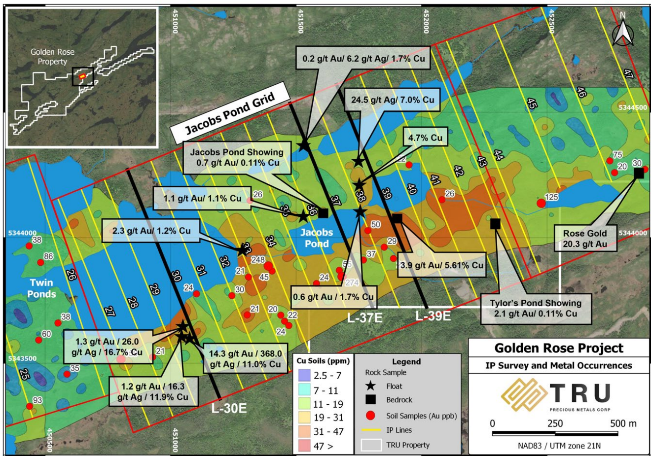
Abb. 1: Planansicht von IP-Linien mit Mineralvorkommen und Kupfer/Gold-in-Boden
