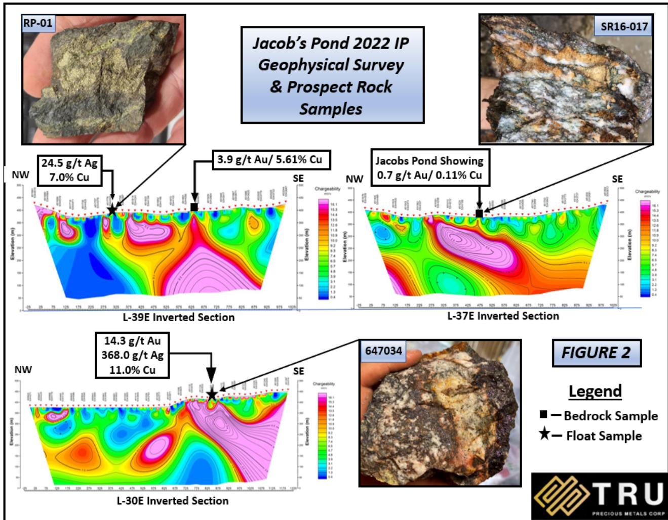
Abb. 2: Ausgewählte IP-Bereiche mit mineralisierten Proben
